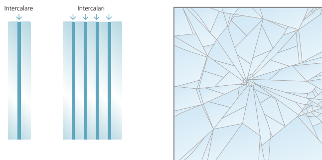
Tipo di frammentazione di un vetro stratificato.
